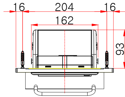
평(윗)면도
