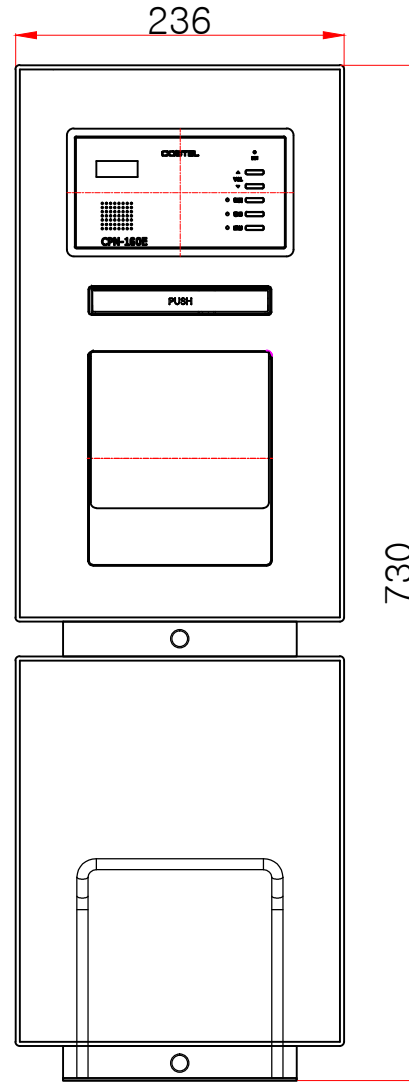
정면도
