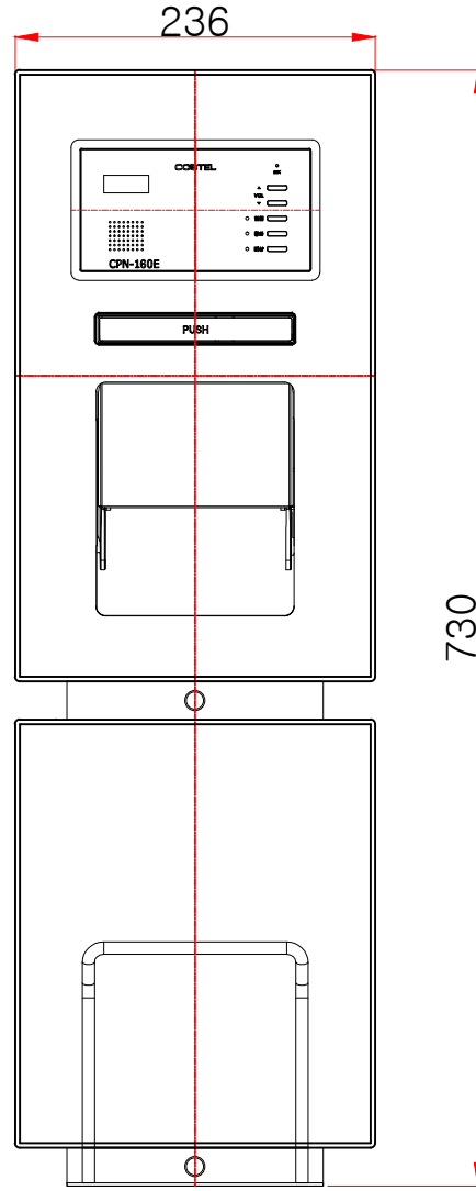
정면도
