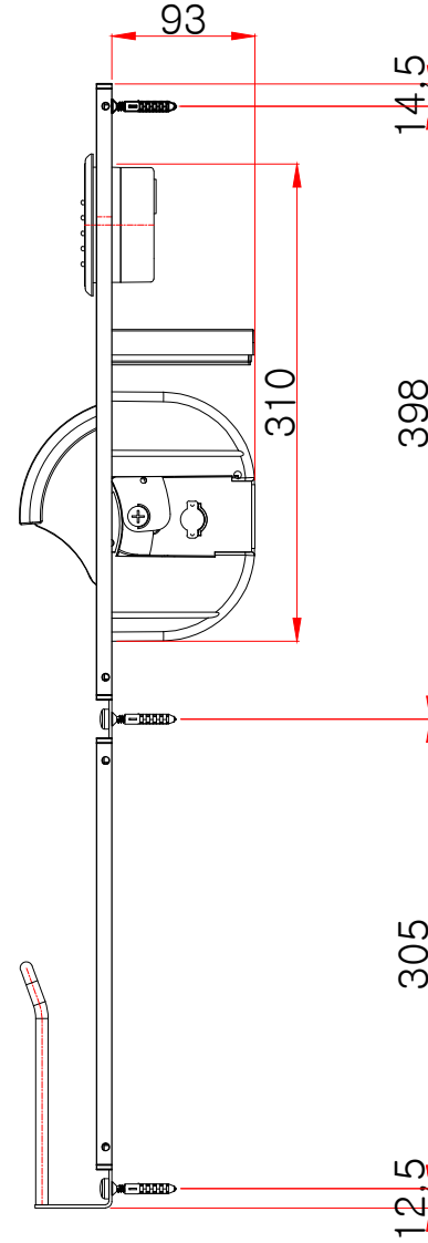
측면도
