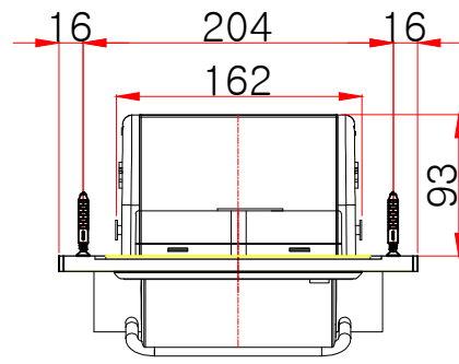
상면도
