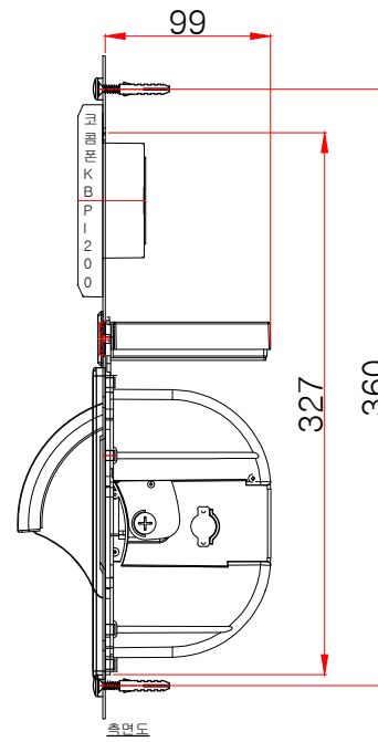
측면도
