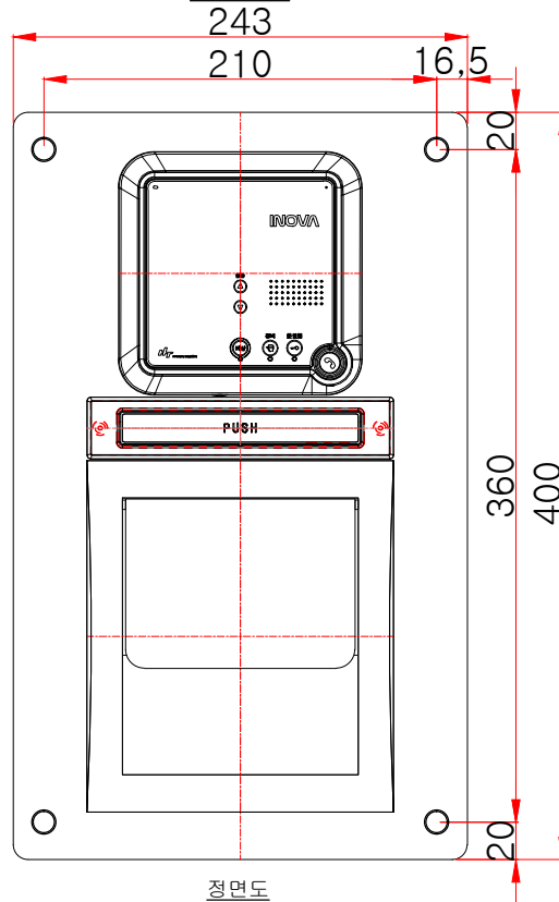
정면도
