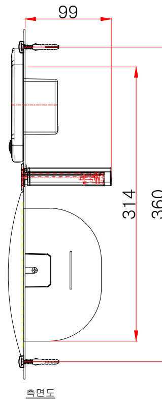
측면도
