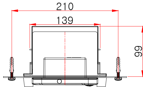
평(윗)면도
