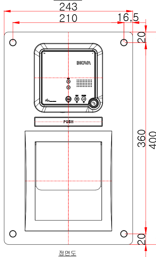
정면도
