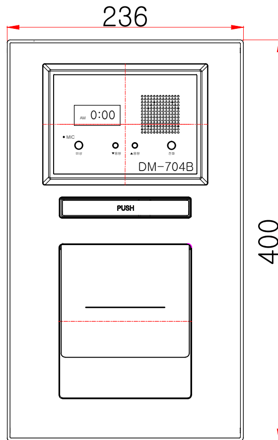
정면도
