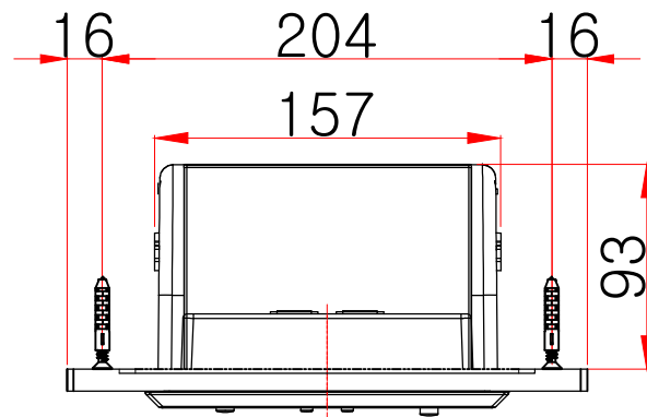
평(윗)면도
