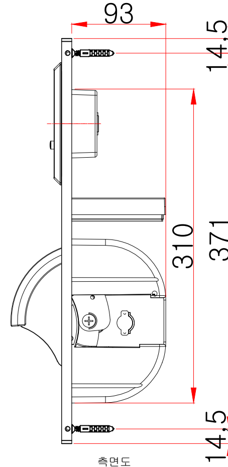
측면도
