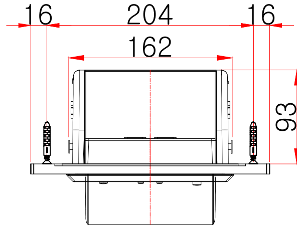
평(위)면도
