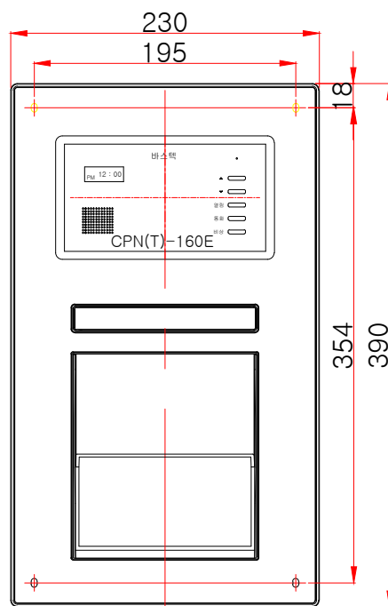
정면도
