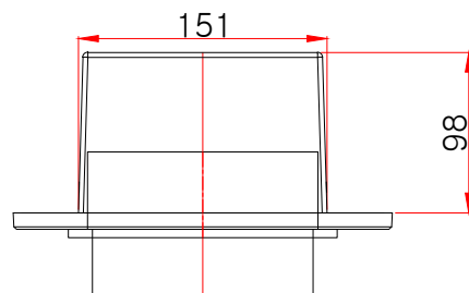
평(윗)면도
