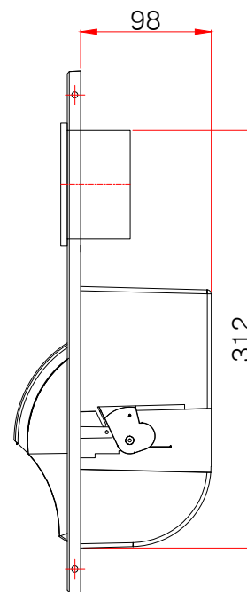
측면도
