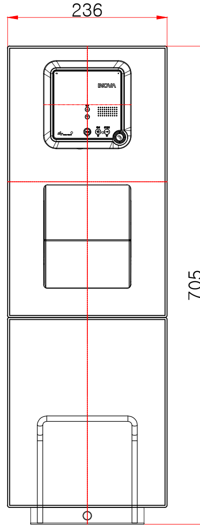
정면도
