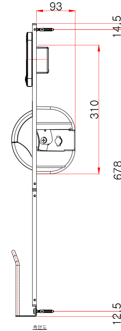
측면도
