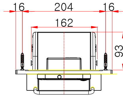
평(위)면도
