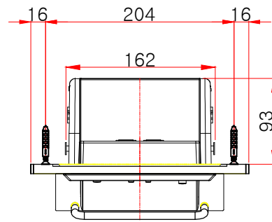
윗면도
