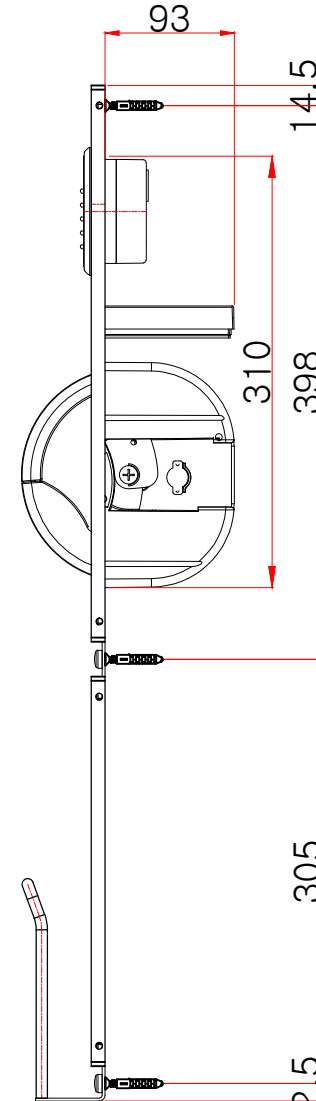
측면도
