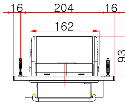
윗면도
