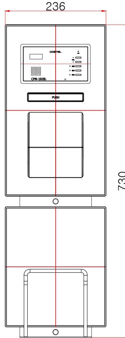
정면도
