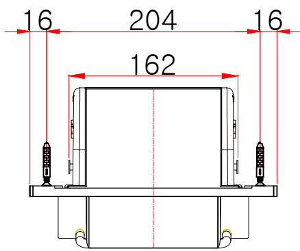
평(윗)면도
