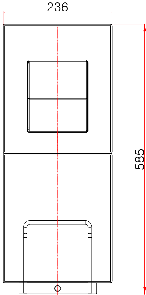
평(윗)면도
