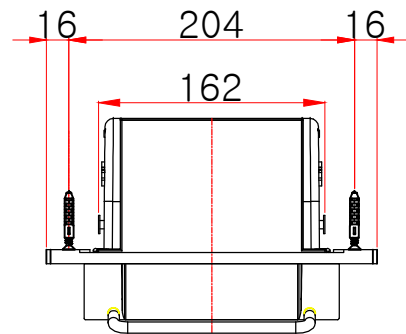
평(위)면도
