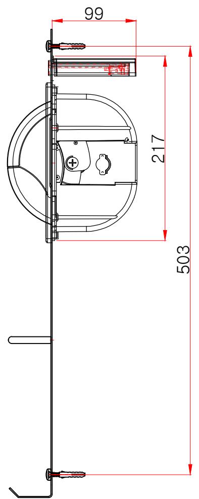
측면도
