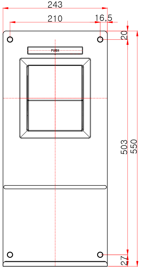
정면도
