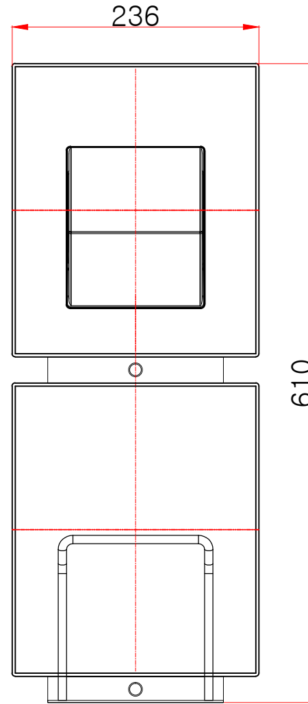
정면도
