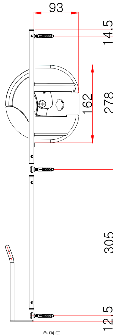
측면도
