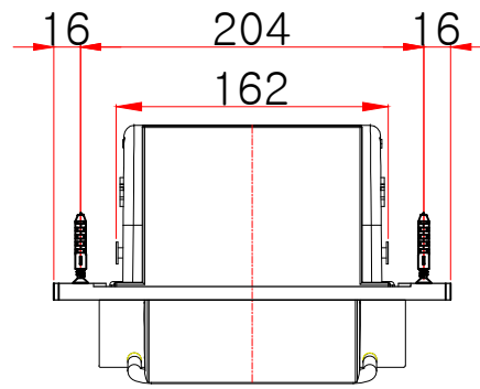
평(윗)면도
