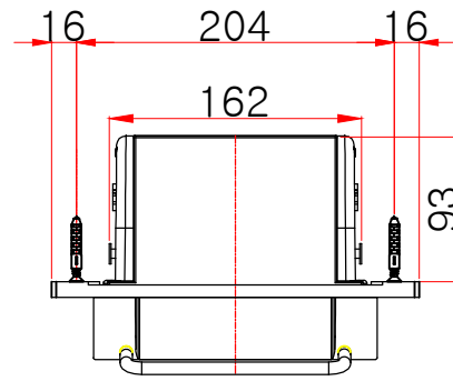
평(위)면도
