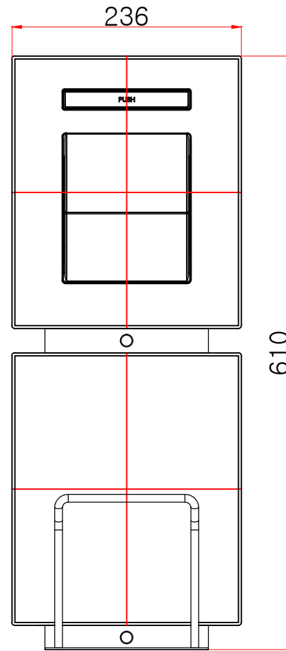
정면도
