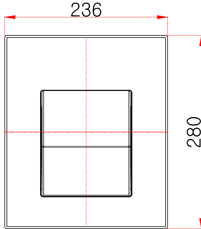
정면도
