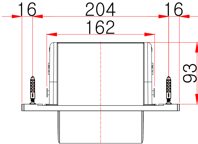
평(윗)면도
