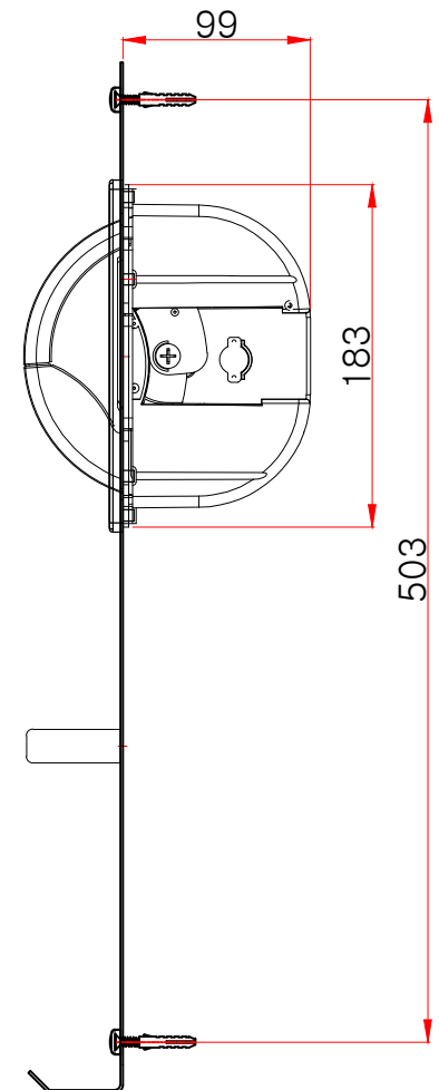
측면도
