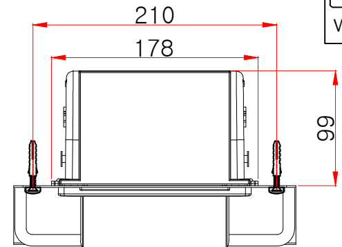
평(위)면도
