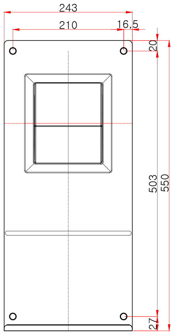
정면도
