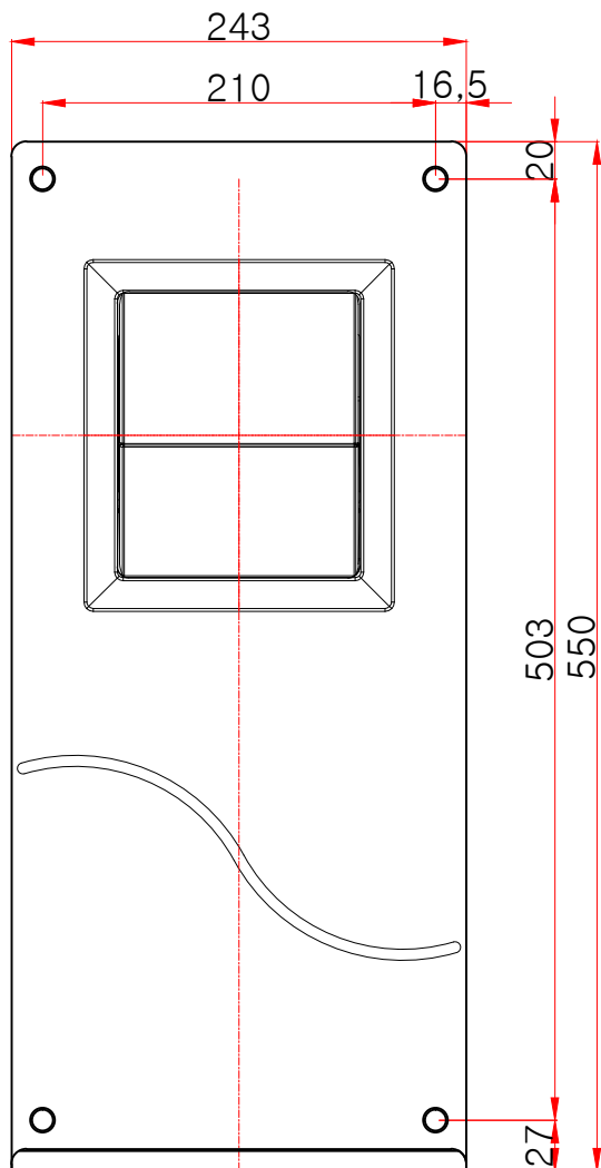
정면도
