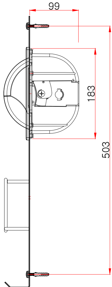
측면도
