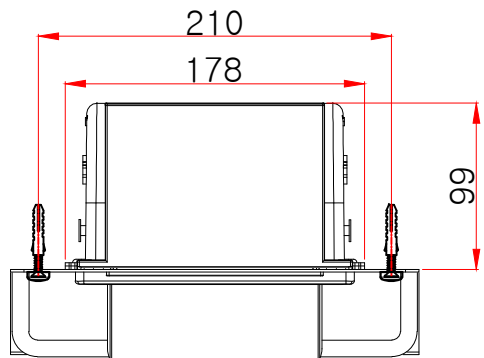
평(위)면도
