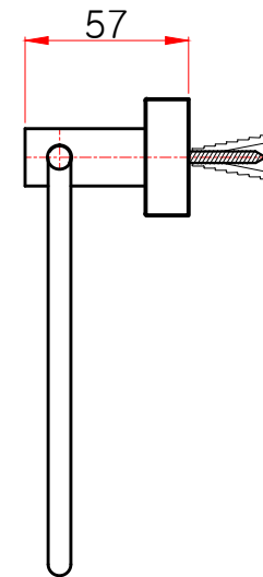
측면도
