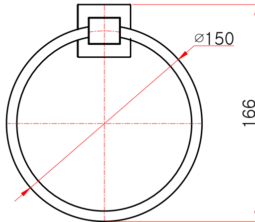
정면도
