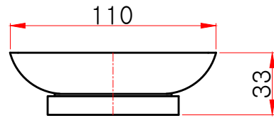
정면도
