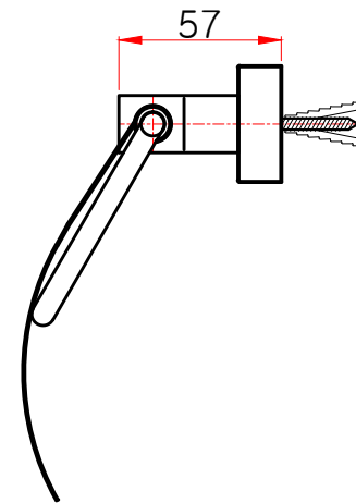
측면도
