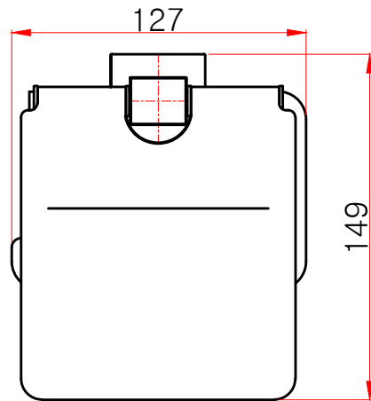
정면도
