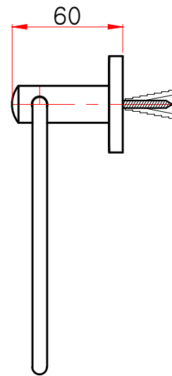
측면도
