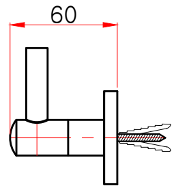
측면도
