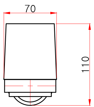
정면도
