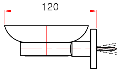
측면도
