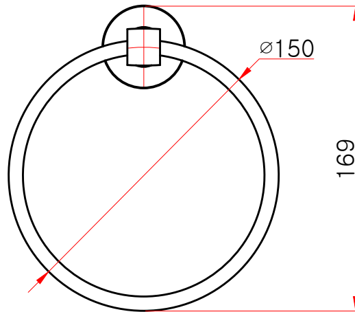
정면도
