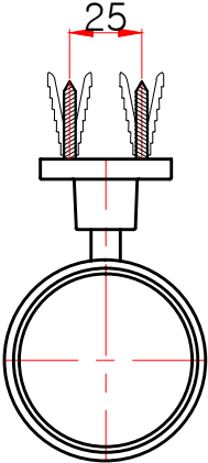
평(윗)면도
