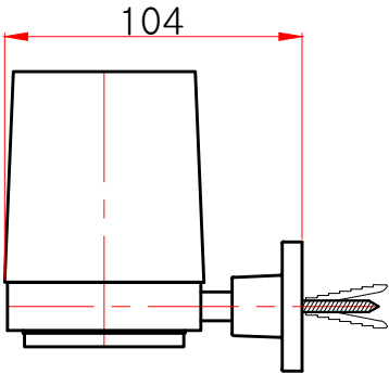
측면도
