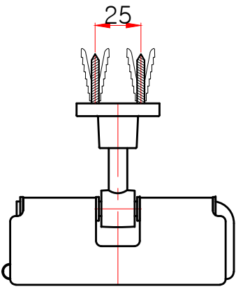
평(윗)면도
