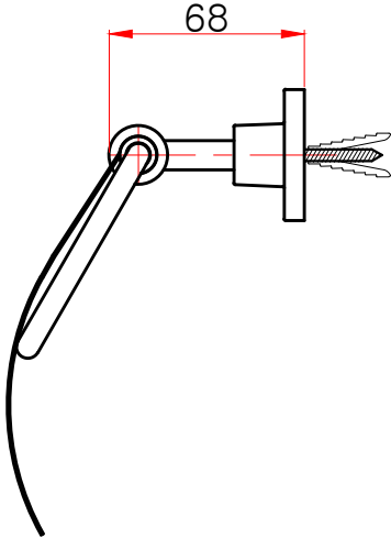
측면도
