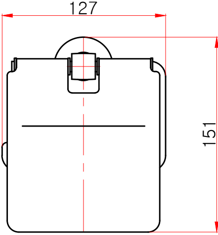
정면도
