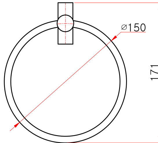
정면도
