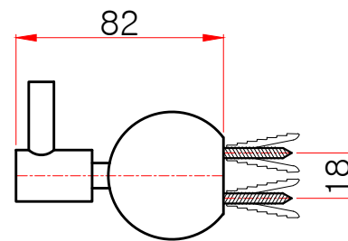
측면도
