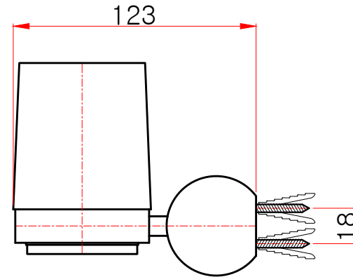
측면도
