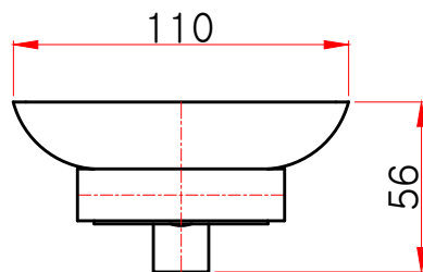
정면도
