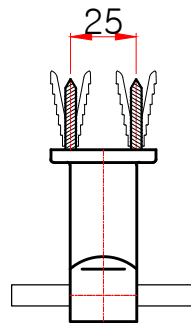
평(윗)면도
