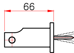
측면도
