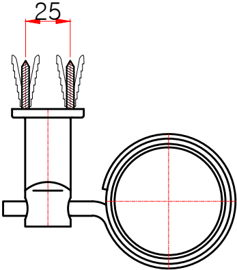
평(윗)면도
