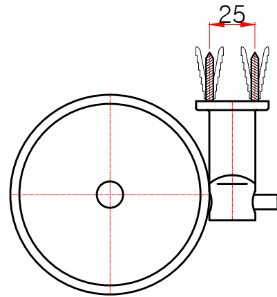
평(윗)면도
