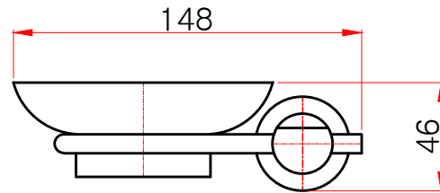
정면도
