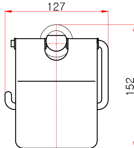
정면도
