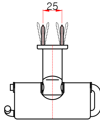
평(윗)면도
