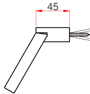
측면도
