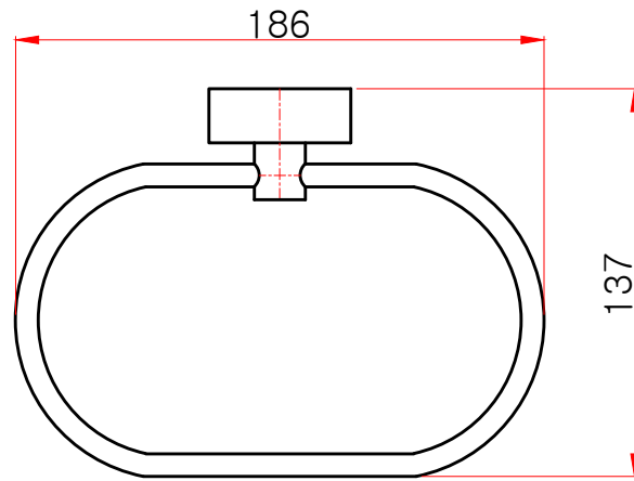
정면도
