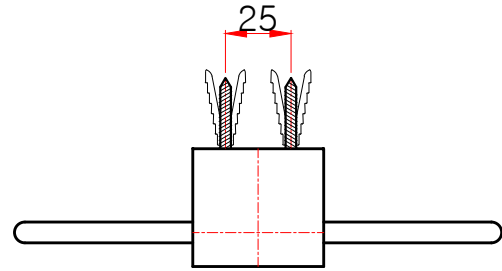
평(윗)면도
