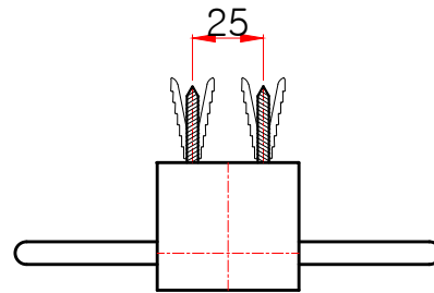
평(윗)면도
