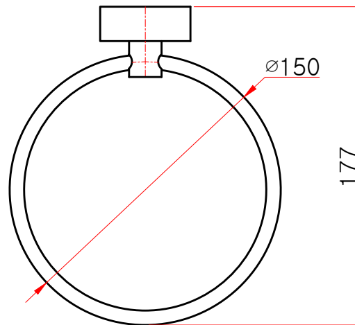
정면도
