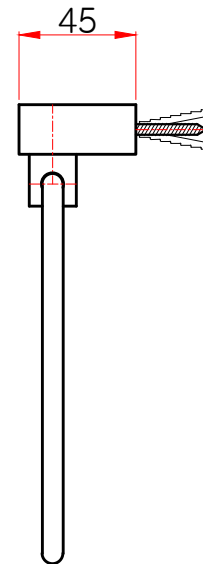
측면도
