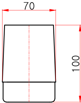
정면도
