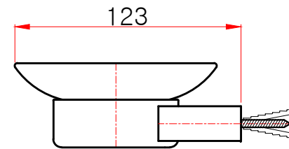
측면도
