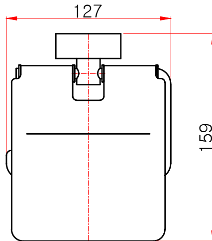
정면도
