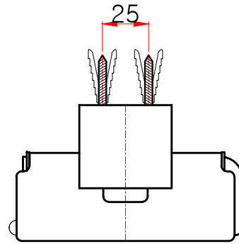
평(윗)면도
