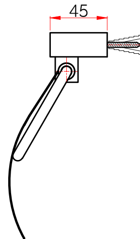
측면도
