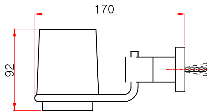
측면도
