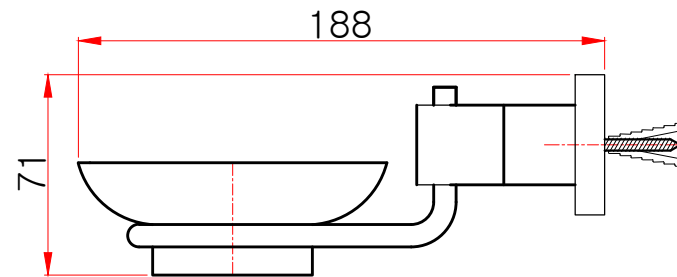
측면도
