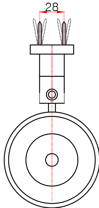
평(윗)면도
