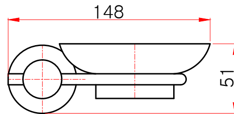
정면도
