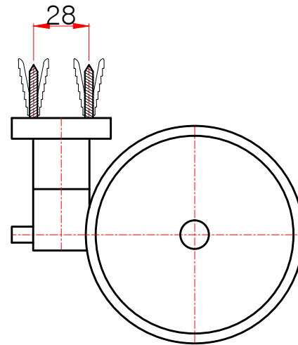
평(윗)면도
