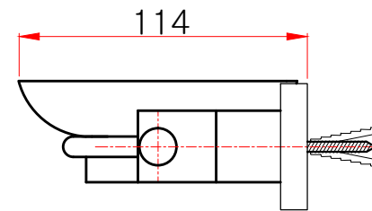
측면도
