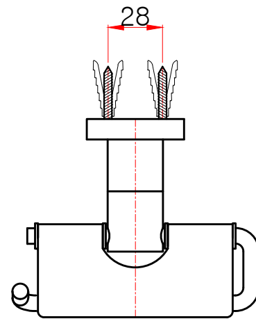
평(윗)면도
