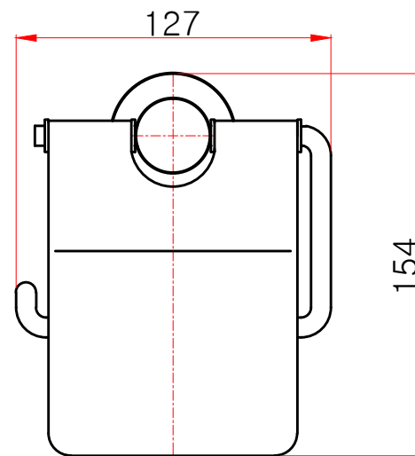
정면도
