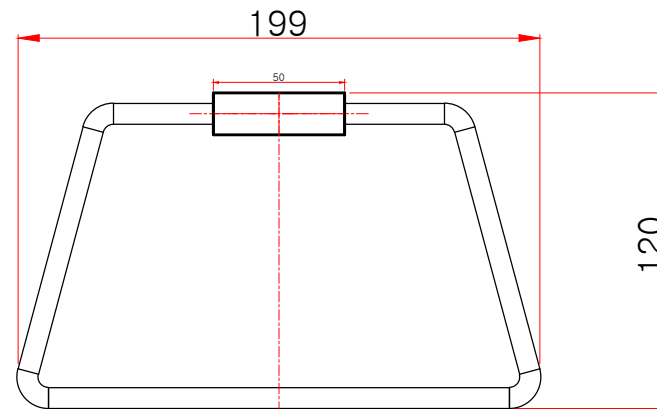
정면도
