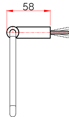
측면도
