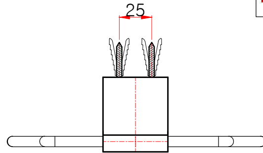
평(윗)면도
