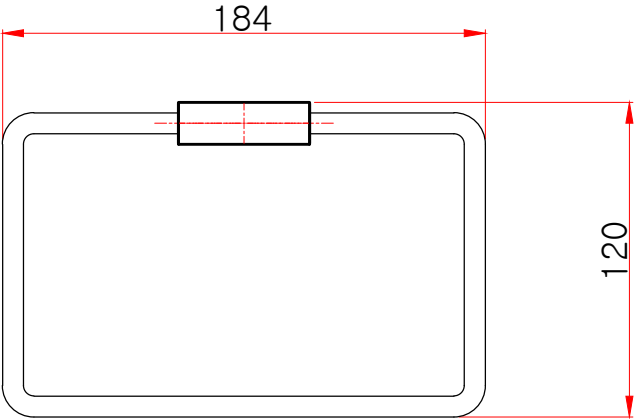
정면도
