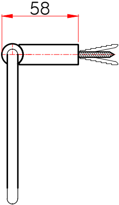
측면도
